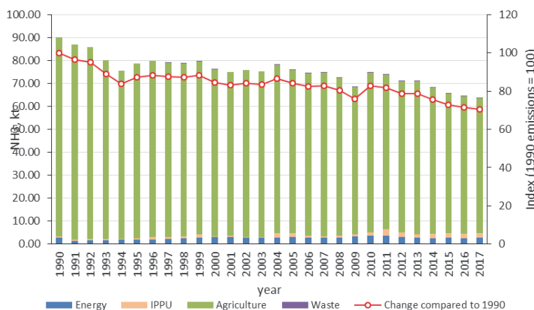
Διάγραμμα 4: Πορεία των εκπομπών \text{NH}_3 από το 1990 έως το 2017
