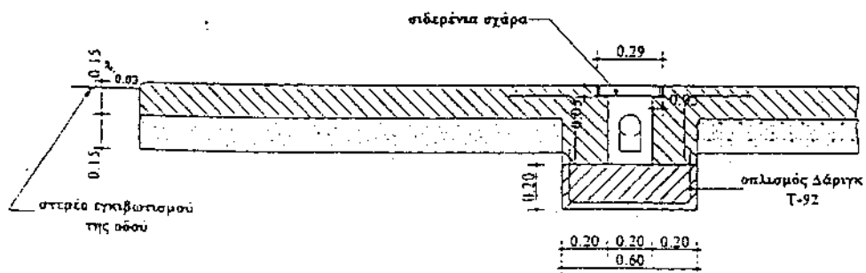
ΤΟΜΗ Β-Β
