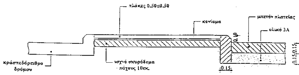
ΤΟΜΗ Α-Α
