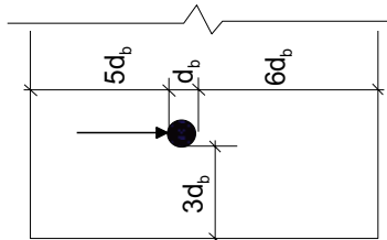
Σχ. Σ6.6: Ορισμός επικάλυψων βλήτρου
