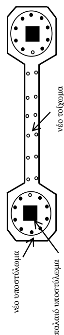
Σχ. Σ8.6: Ενδεικτική εμφάνωση με πάχος ίσο ή μικρότερο του πλάτους της δοκού
